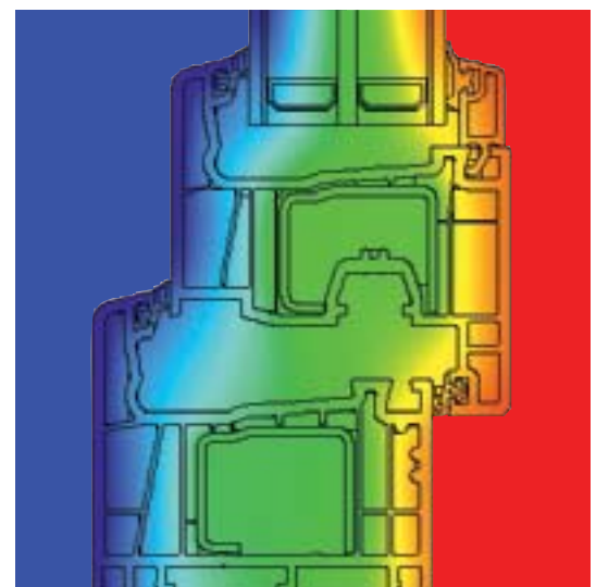
Wärmeisoliertes Fenster: Das Temperaturbild zeigt den Verlauf der Isothermen
